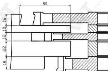
Блок 11. Коробковий шип Блок 11. Коробочный шип Block 11. Box spike
