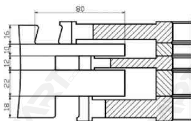
Блок 9. Стулка-шипи Блок 9. Створка-шипы Block 9. Door-spikes
