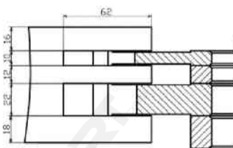
Блок 10. Стулка-вушко Блок 10. Створка-ушко Block 10. Door-ear
