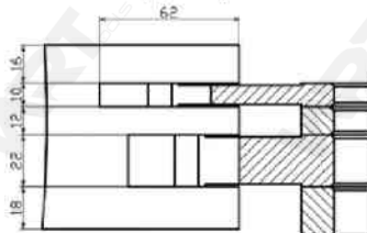
Блок 12. Коробка вушко верхнє Блок 12. Коробка ушко верхнє Block 12. Upper eyelet box
